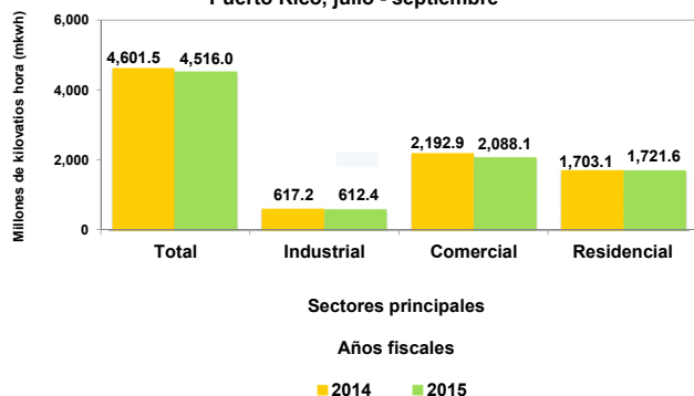
Gráfica 5: Consumo de energía eléctrica total y por sectores principales Puerto Rico, julio - septiembre
