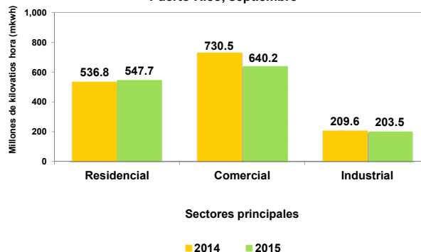
Gráfica 4: Consumo de energía eléctrica por sectores principales Puerto Rico, septiembre
