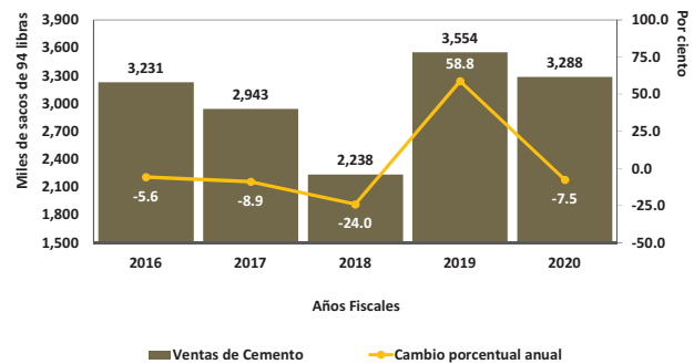
Gráfica 2: Ventas de Cemento (Cambio porcentual anual, período de julio a septiembre)
