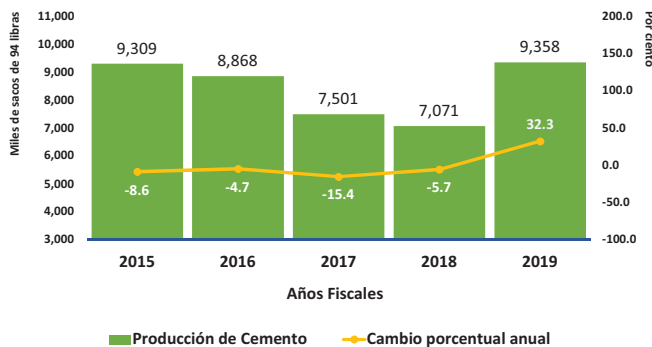
Gráfica 1: Producción de Cemento (Cambio porcentual anual, período de julio a marzo)
