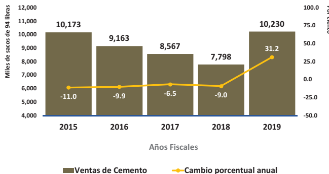
Gráfica 2: Ventas de Cemento (Cambio porcentual anual, período de julio a marzo)
