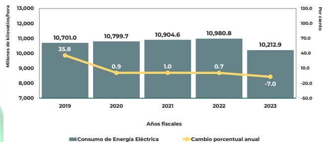
Gráfica 2: Consumo de Energía Eléctrica (Cambio porcentual anual, período de julio a febrero)
