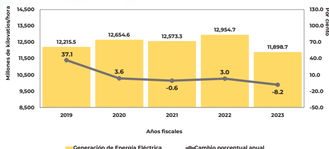
Gráfica 1: Generación de Energía Eléctrica (Cambio porcentual anual, período de julio a febrero)
