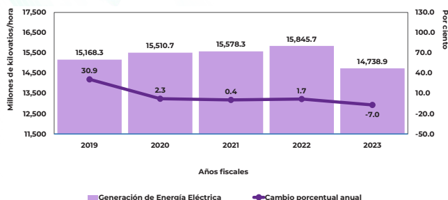
Gráfica 1: Generación de Energía Eléctrica (Cambio porcentual anual, período de julio a abril)
